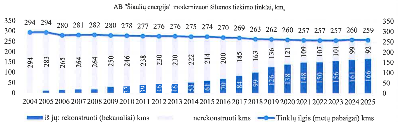
6 pav. AB „Šiaulių energija“ modernizuoti šilumos tinklai
