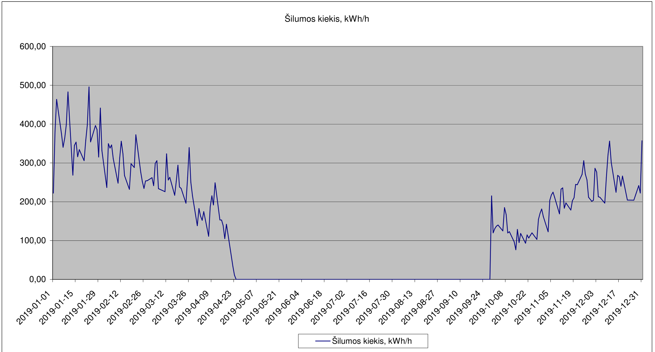
2019 m. Ventos katilinės paros vidutinės šilumos gamybos grafikas
