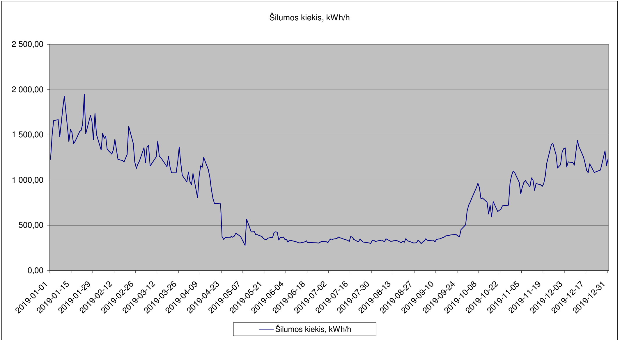
2019 m. Stumbro katilinės paros vidutinės šilumos gamybos grafikas
