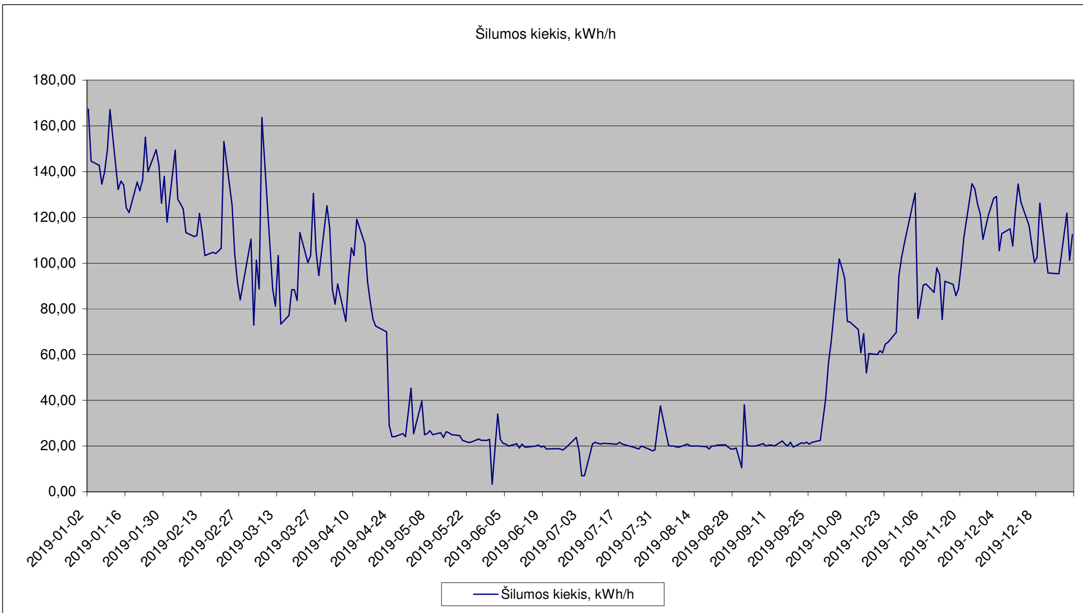
2019 m. Sodo g. katilinės paros vidutinės šilumos gamybos grafikas
