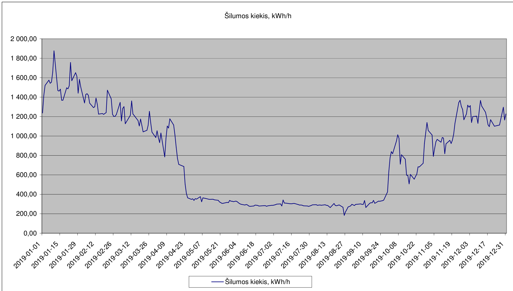
2019 m. Rėkyvos katilinės paros vidutinės šilumos gamybos grafikas
