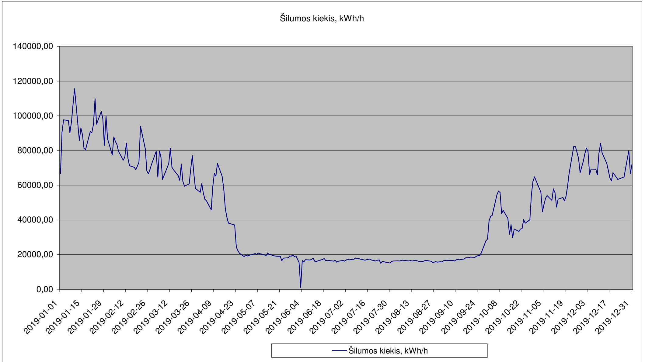
2019 m. Pietinės katilinės ir TE paros vidutinės šilumos gamybos grafikas
