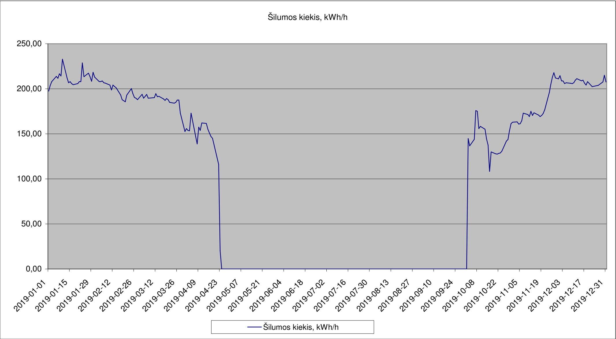
2019 m. Pavenčių katilinės paros vidutinės šilumos gamybos grafikas
