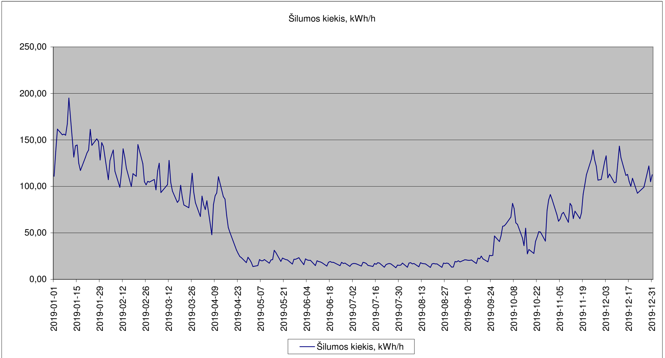
2019 m. Papilės katilinės paros vidutinės šilumos gamybos grafikas
