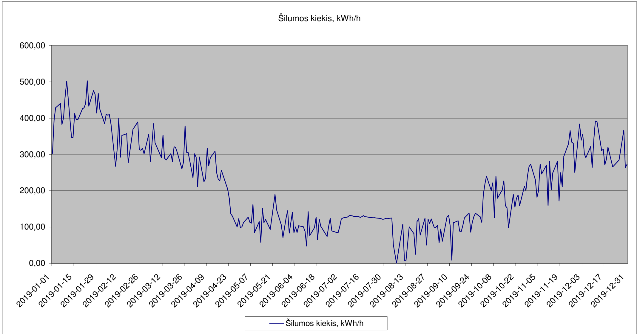
2019 m. Kairių katilinės paros vidutinės šilumos gamybos grafikas
