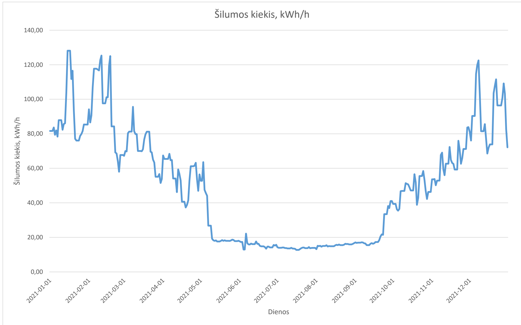
2021m. Pietinės katilinės ir TE paros vidutinės šilumos gamybos grafikas
