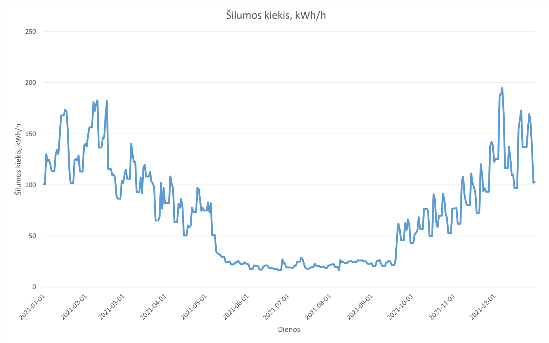
2021m. Papilės katilinės paros vidutinės šilumos gamybos grafikas
