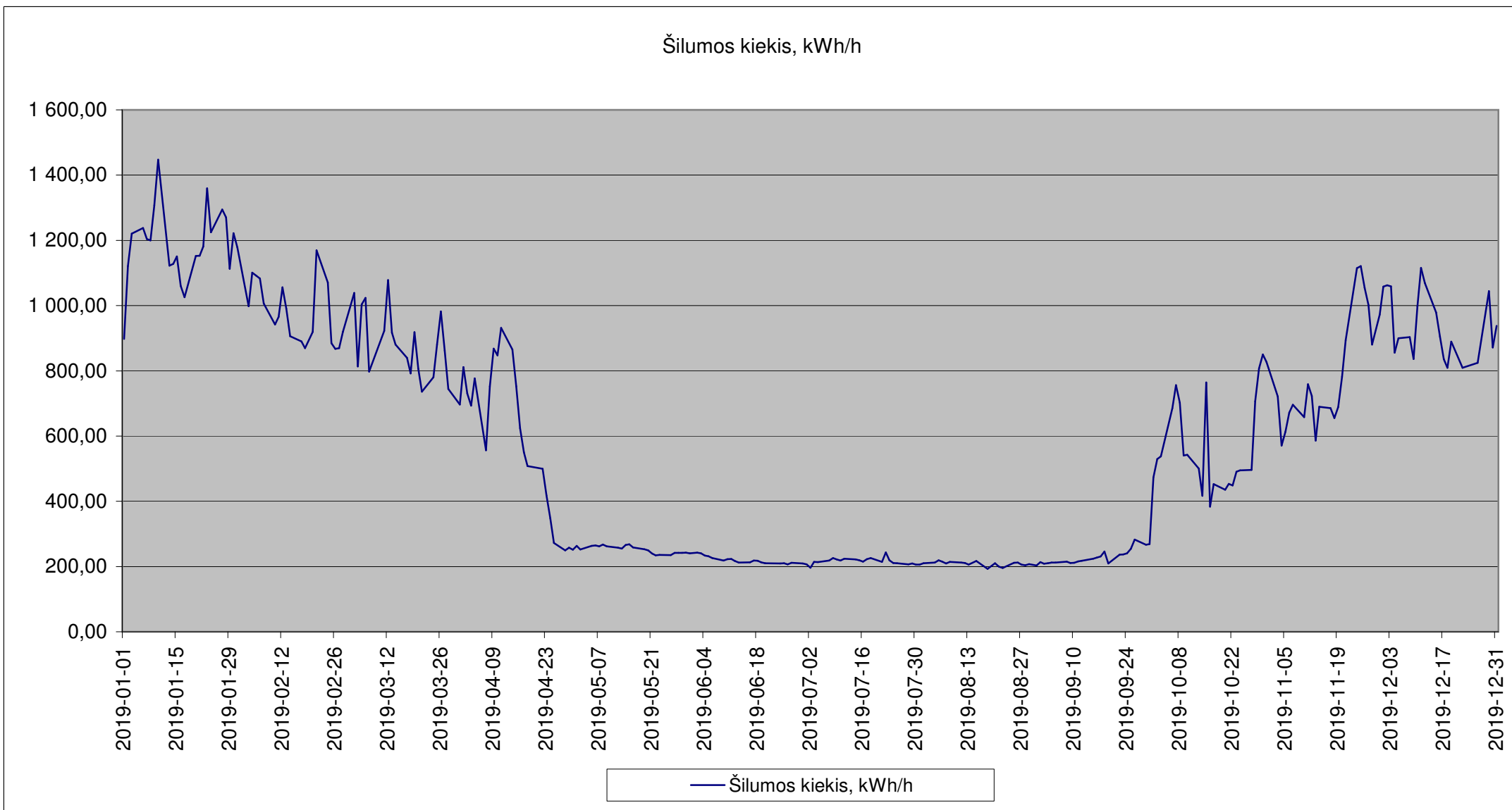
2019 m. Ginkūnų katilinės paros vidutinės šilumos gamybos grafikas
