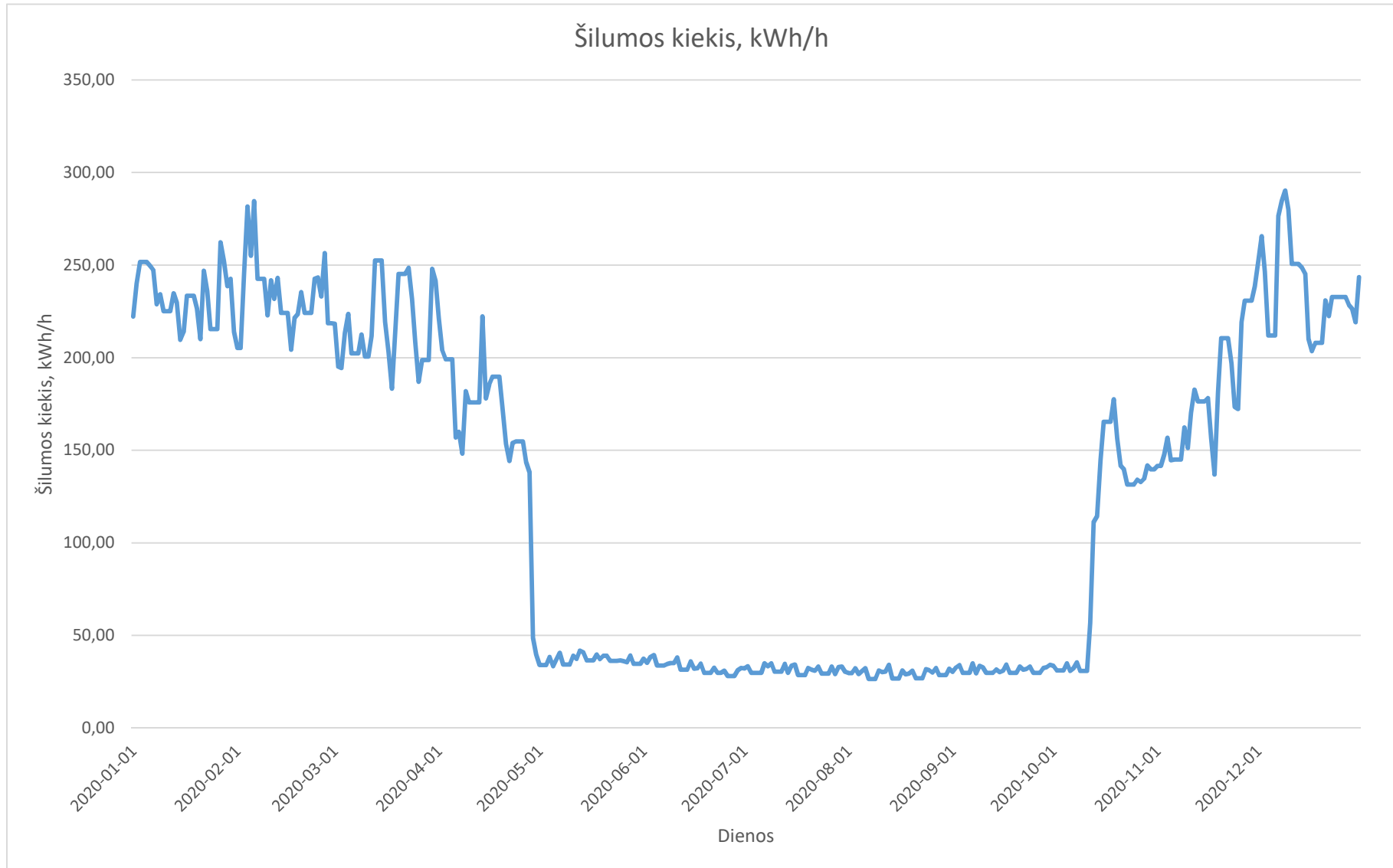
2020 m. Aukštėlkės katilinės paros vidutinės šilumos gamybos grafikas
