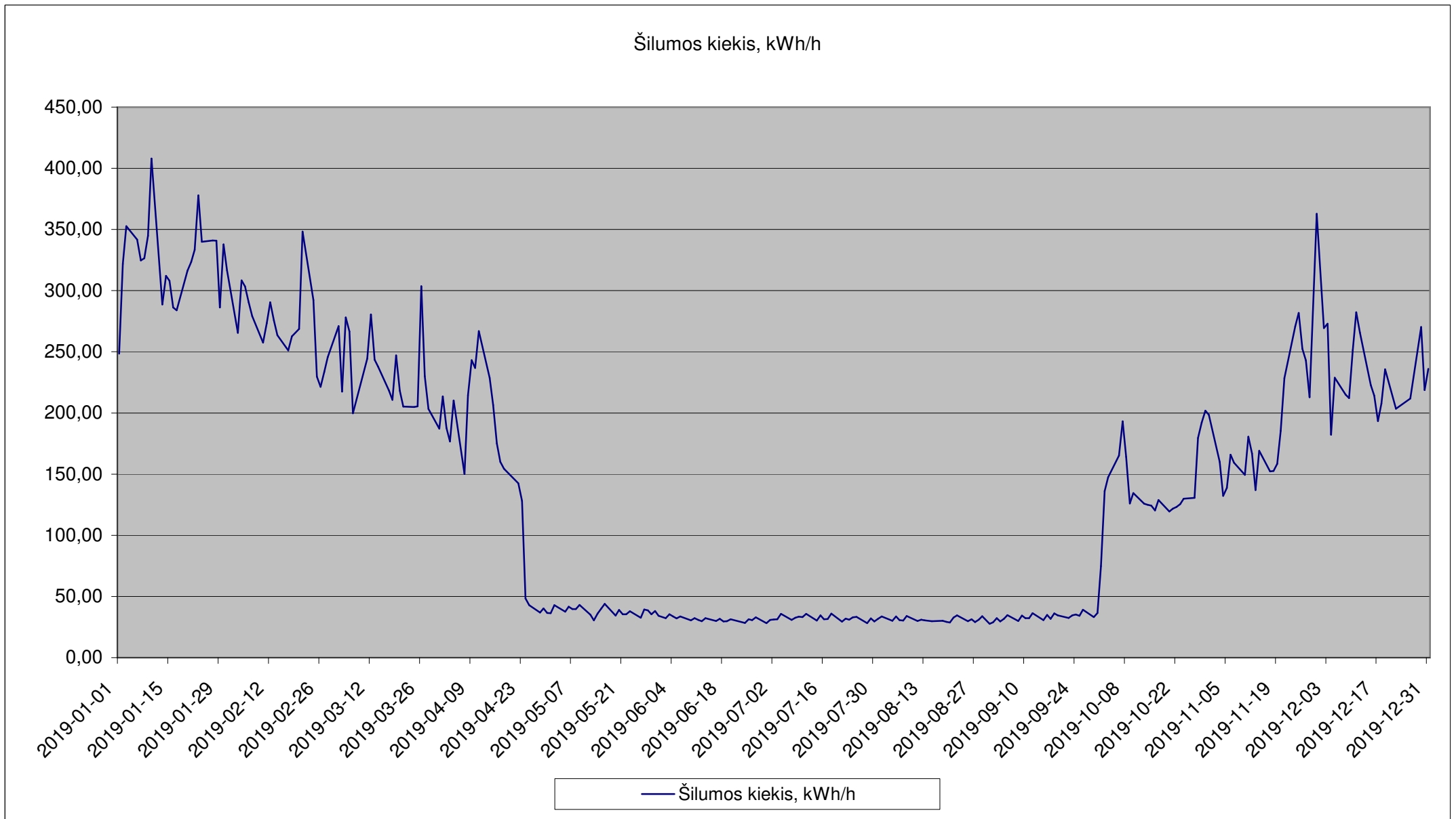
2019 m. Aukštėlkės katilinės paros vidutinės šilumos gamybos grafikas
