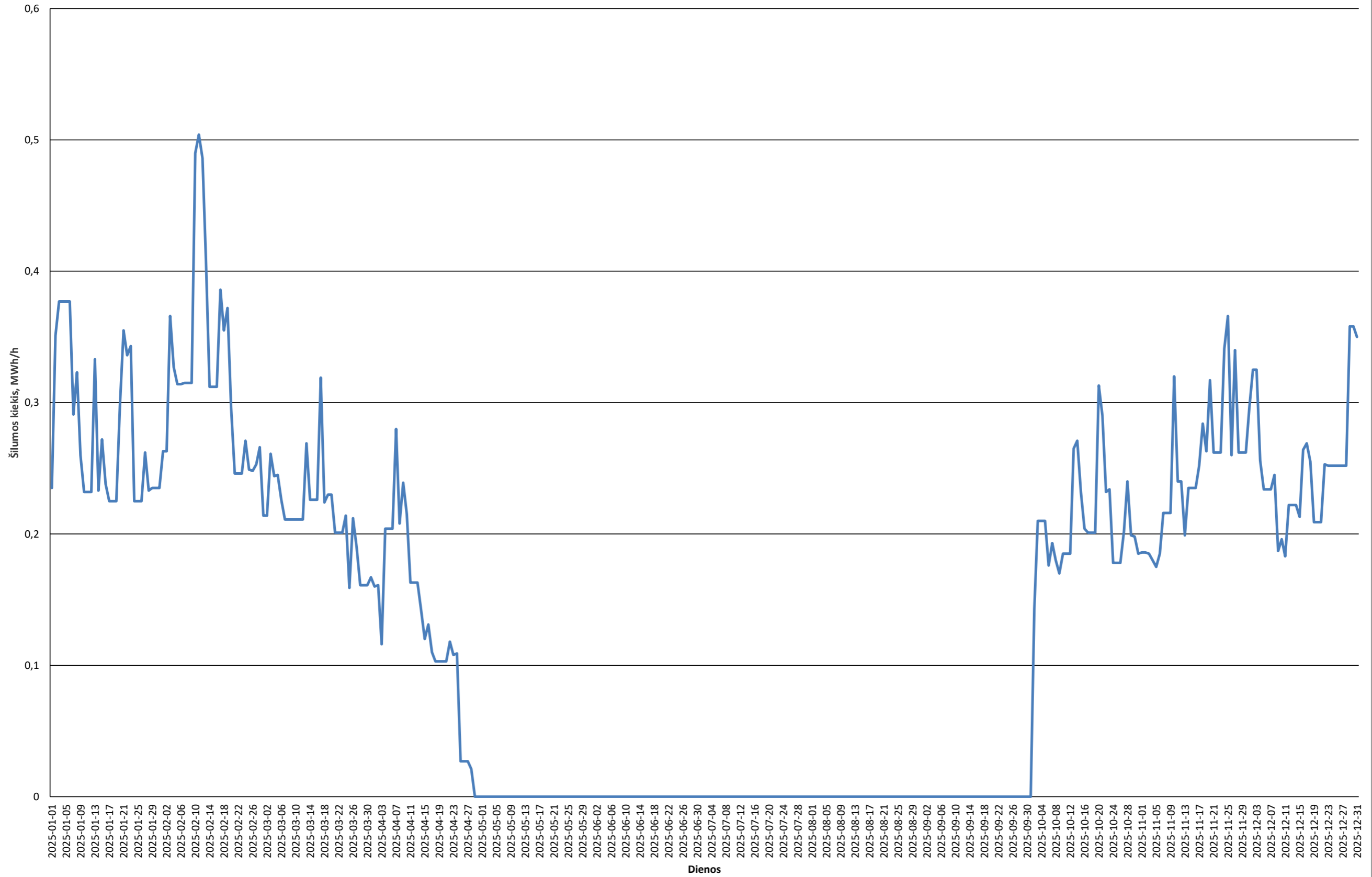
2025 m. Ventos katilinės paros vidutinės šilumos gamybos grafikas
