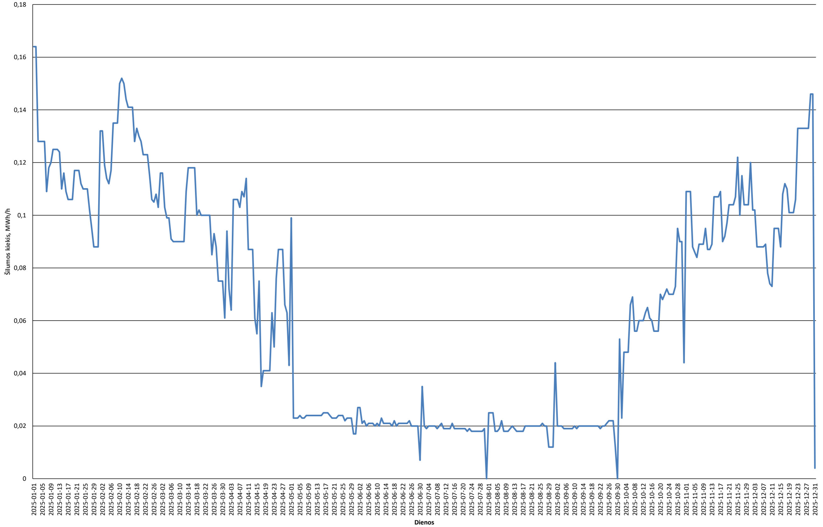
2025 m. Sodo g. katilinės paros vidutinės šilumos gamybos grafikas
