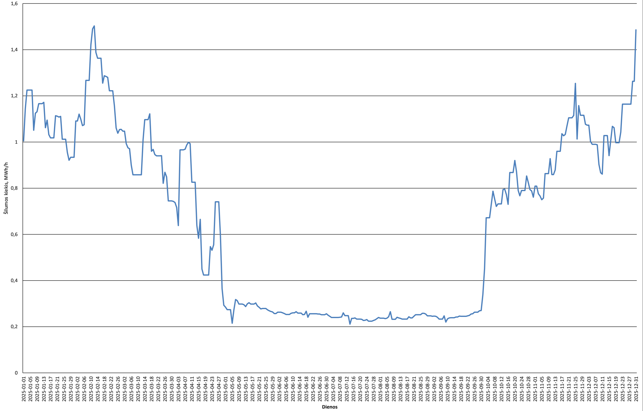
2025 m. Rėkyvos katilinės paros vidutinės šilumos gamybos grafikas
