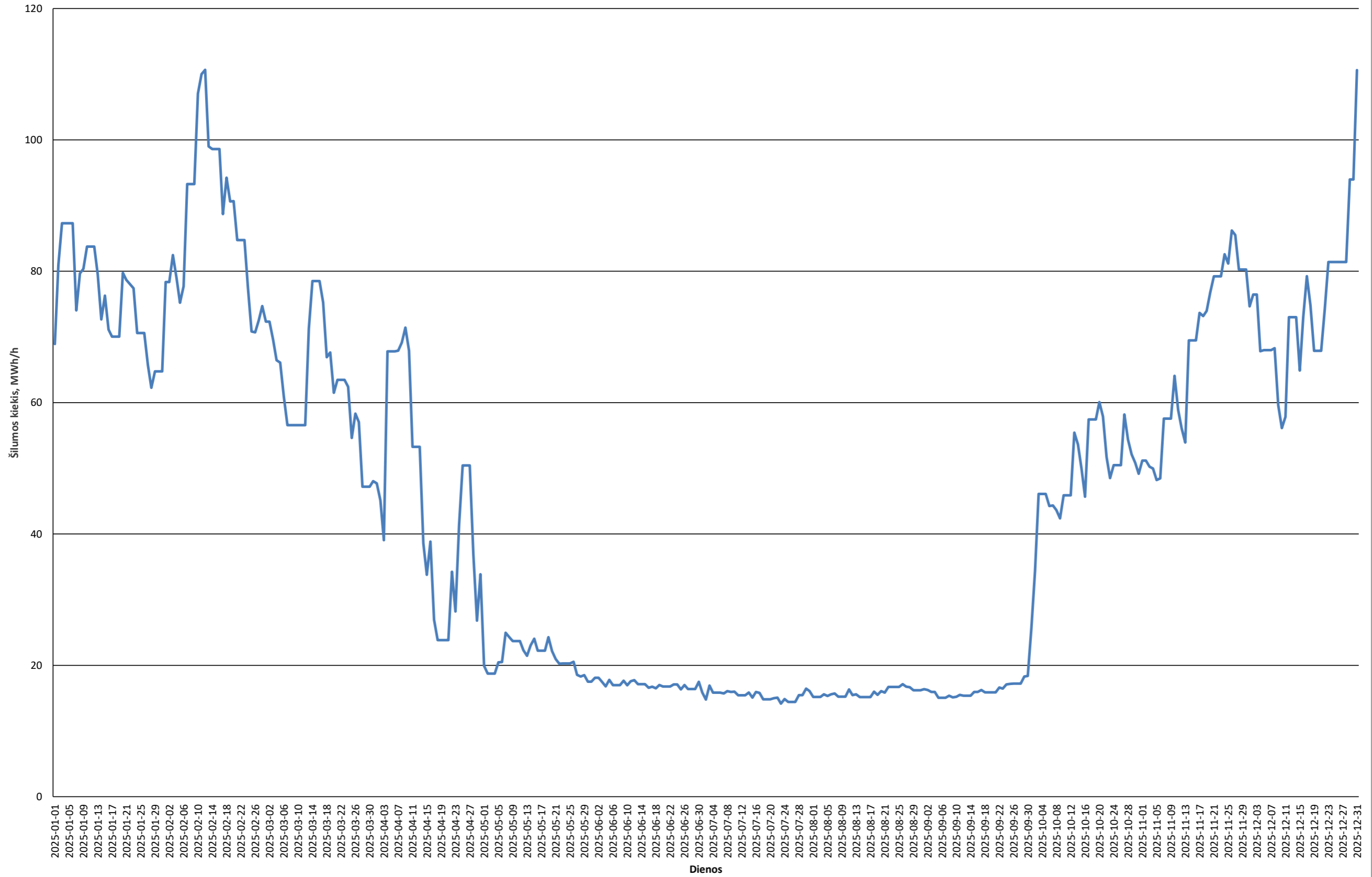
2025 m. Pietinės katilinės paros vidutinės šilumos gamybos grafikas
