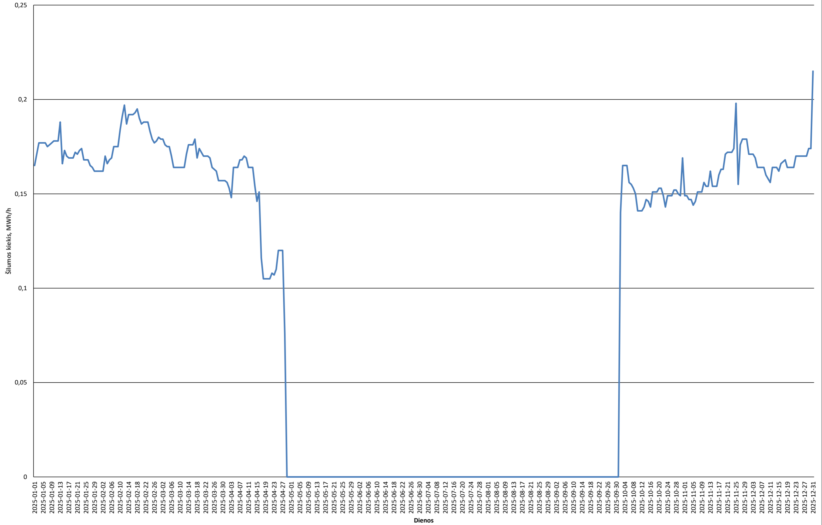
2025 m. Pavenčių katilinės paros vidutinės šilumos gamybos grafikas
