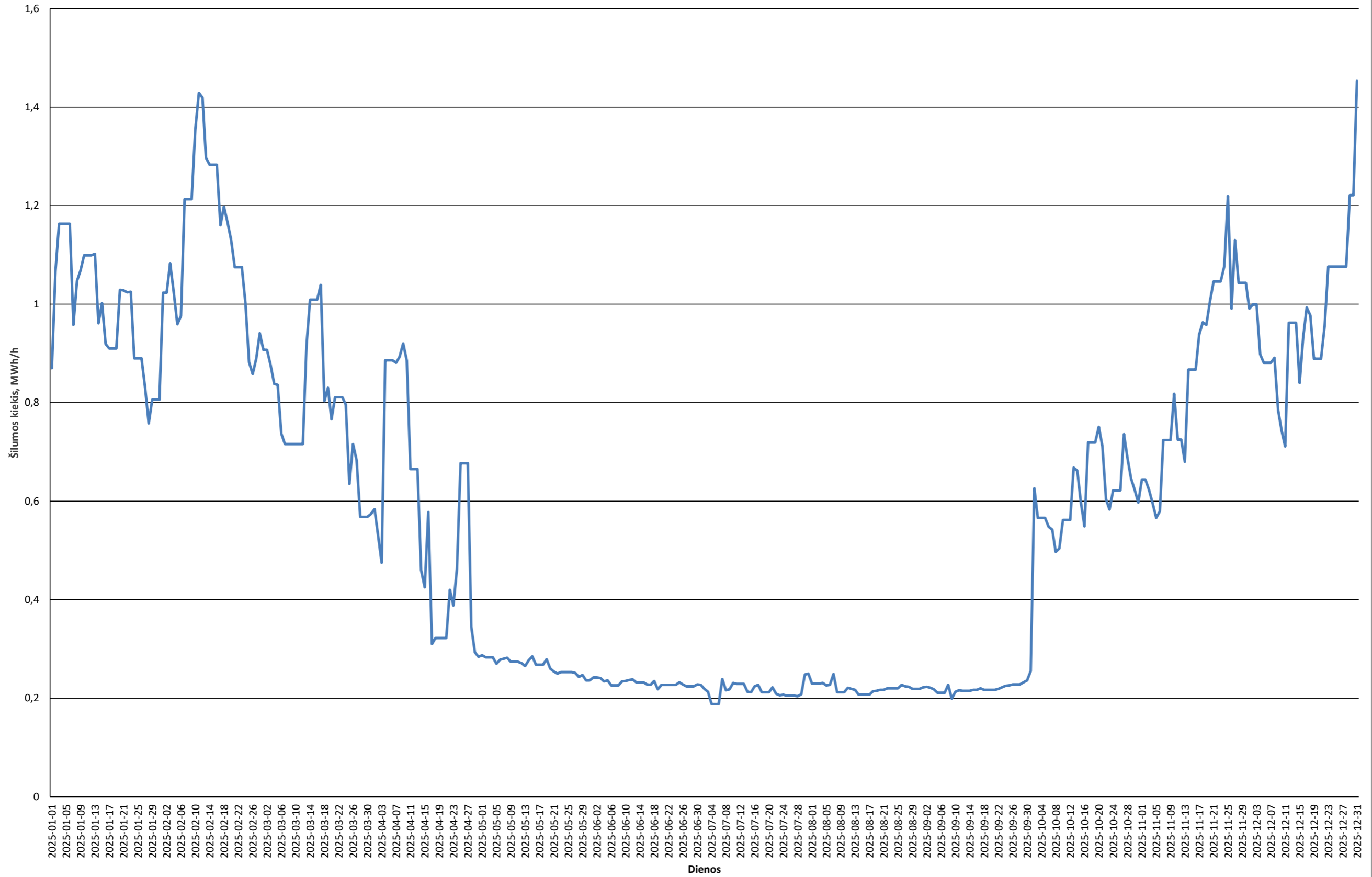
2025 m. Ginkūnų katilinės paros vidutinės šilumos gamybos grafikas
