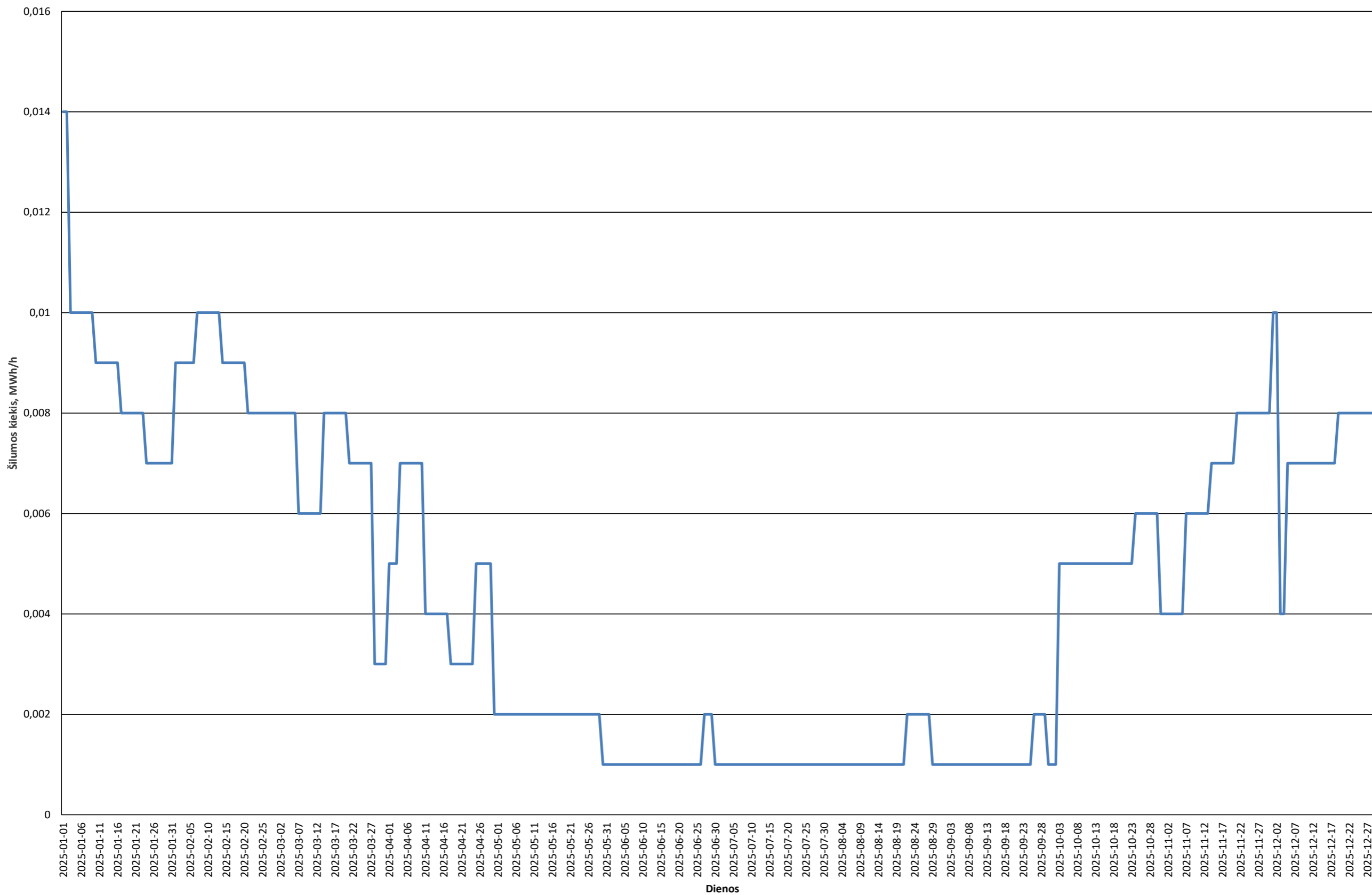
2025 m. J. Basanavičiaus g. 103B katilinės paros vidutinės šilumos gamybos grafikas
