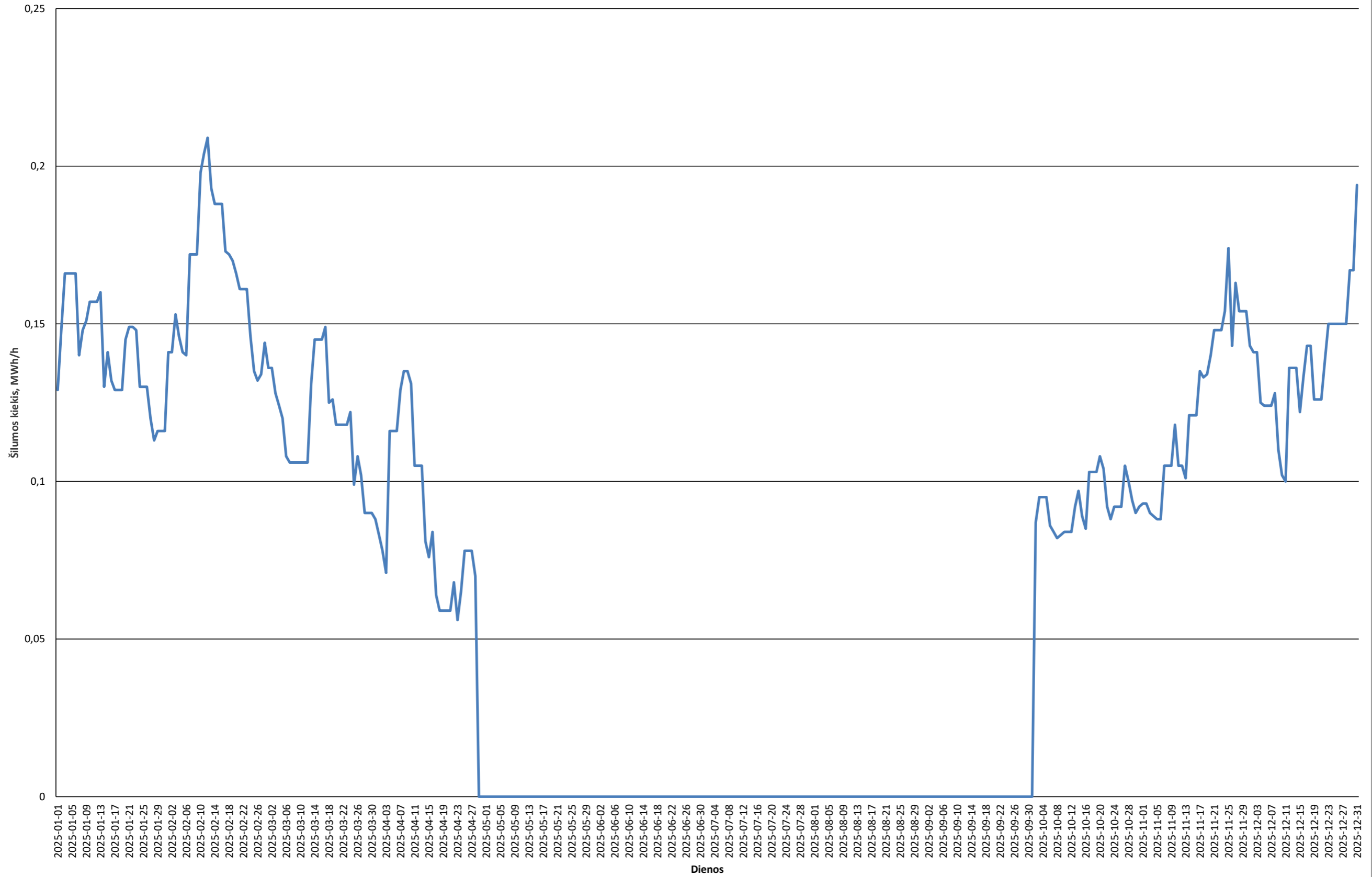
2025 m. Šilėnų katilinės paros vidutinės šilumos gamybos grafikas
