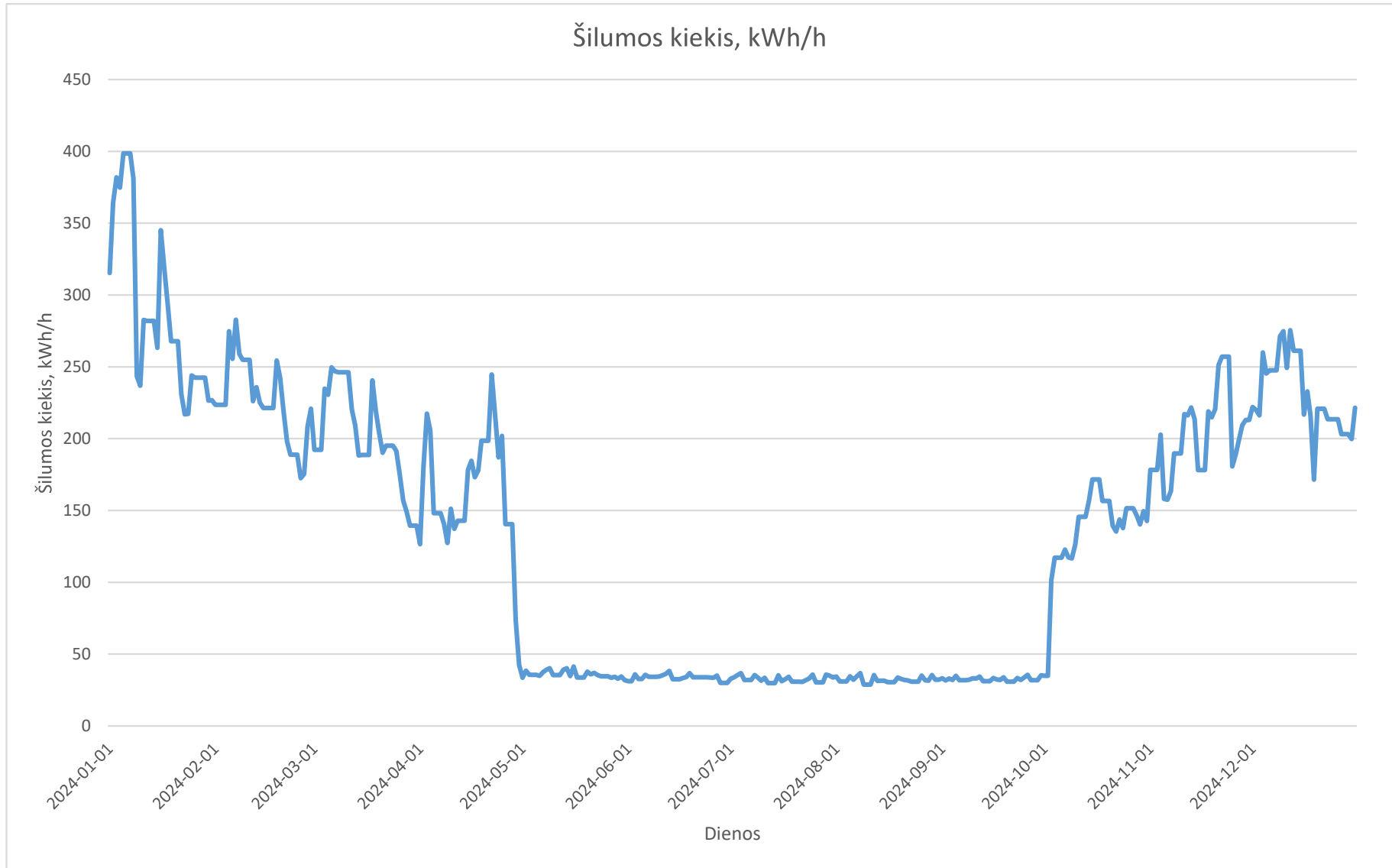
2024m. Aukštelkės katilinės paros vidutinės šilumos gamybos grafikas
