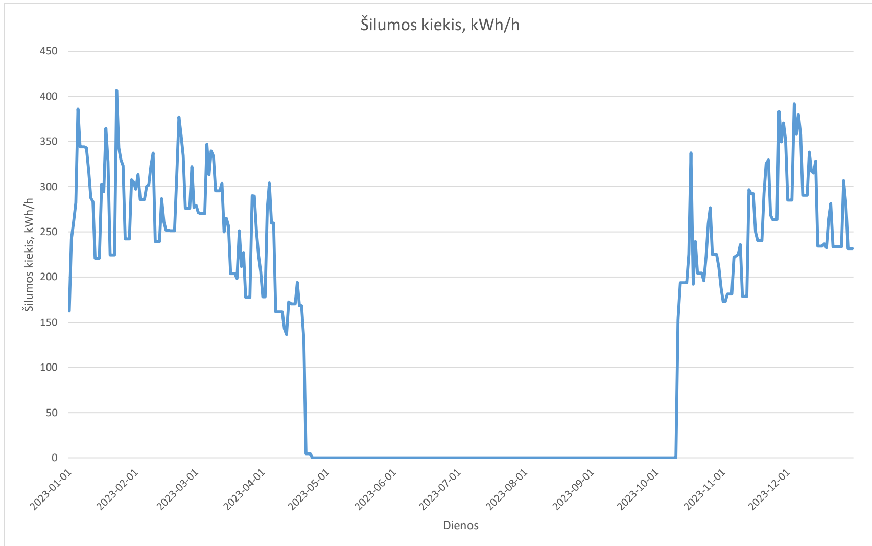
2023m. Ventos katilinės paros vidutinės šilumos gamybos grafikas
