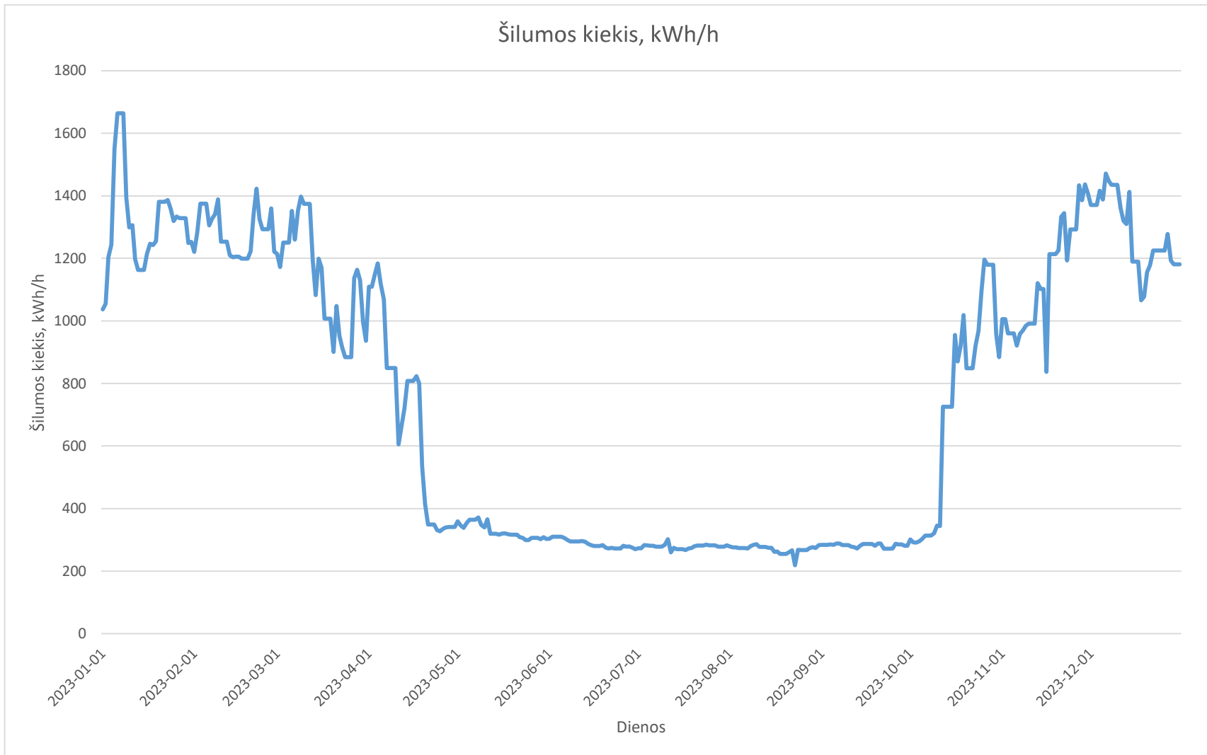
2023m. Rėkyvos katilinės paros vidutinės šilumos gamybos grafikas
