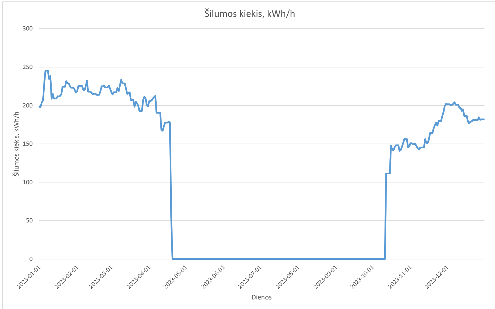
2023m. Pavenčių katilinės paros vidutinės šilumos gamybos grafikas
