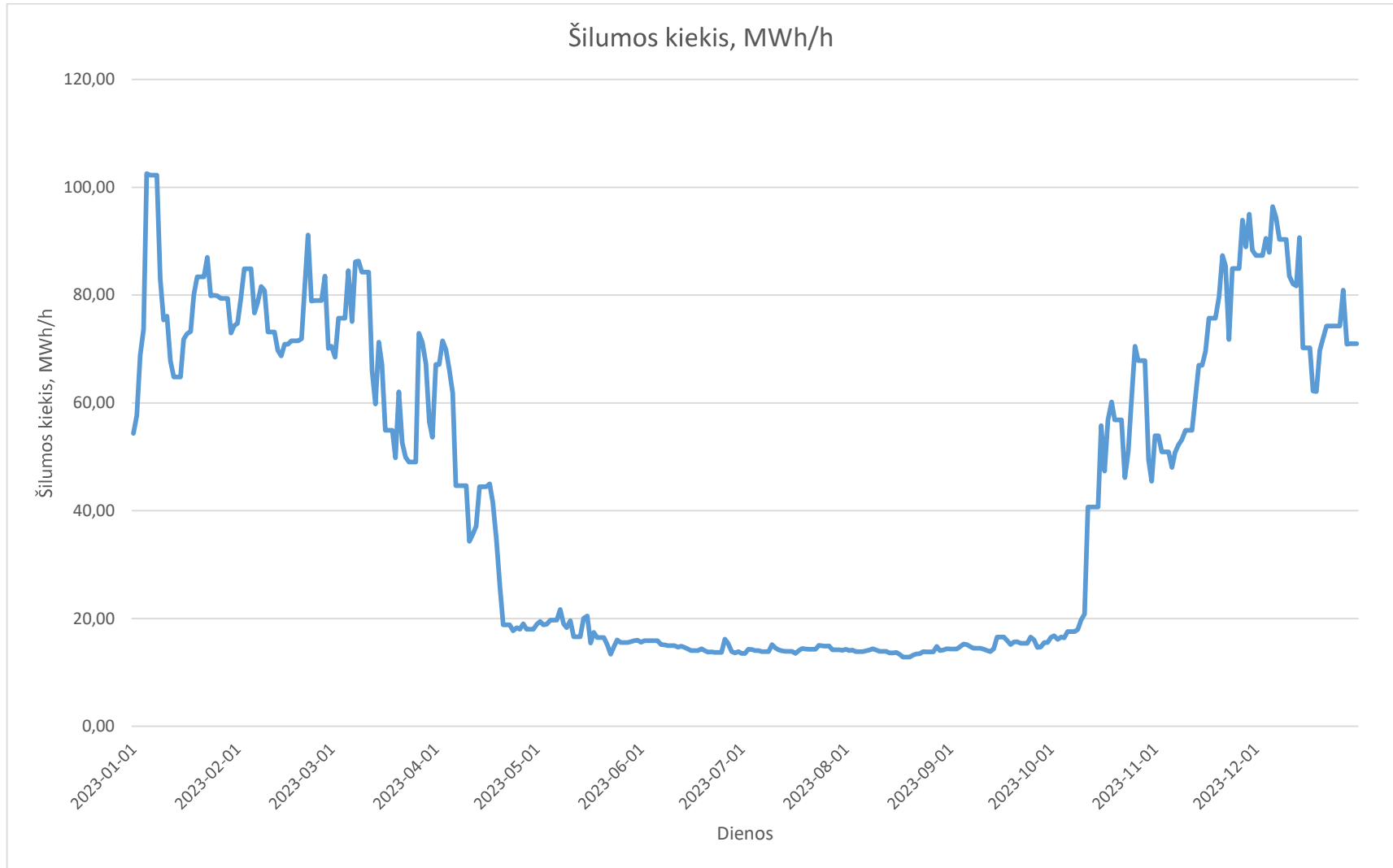
2023m. Pietinės katilinės ir TE paros vidutinės šilumos gamybos grafikas
