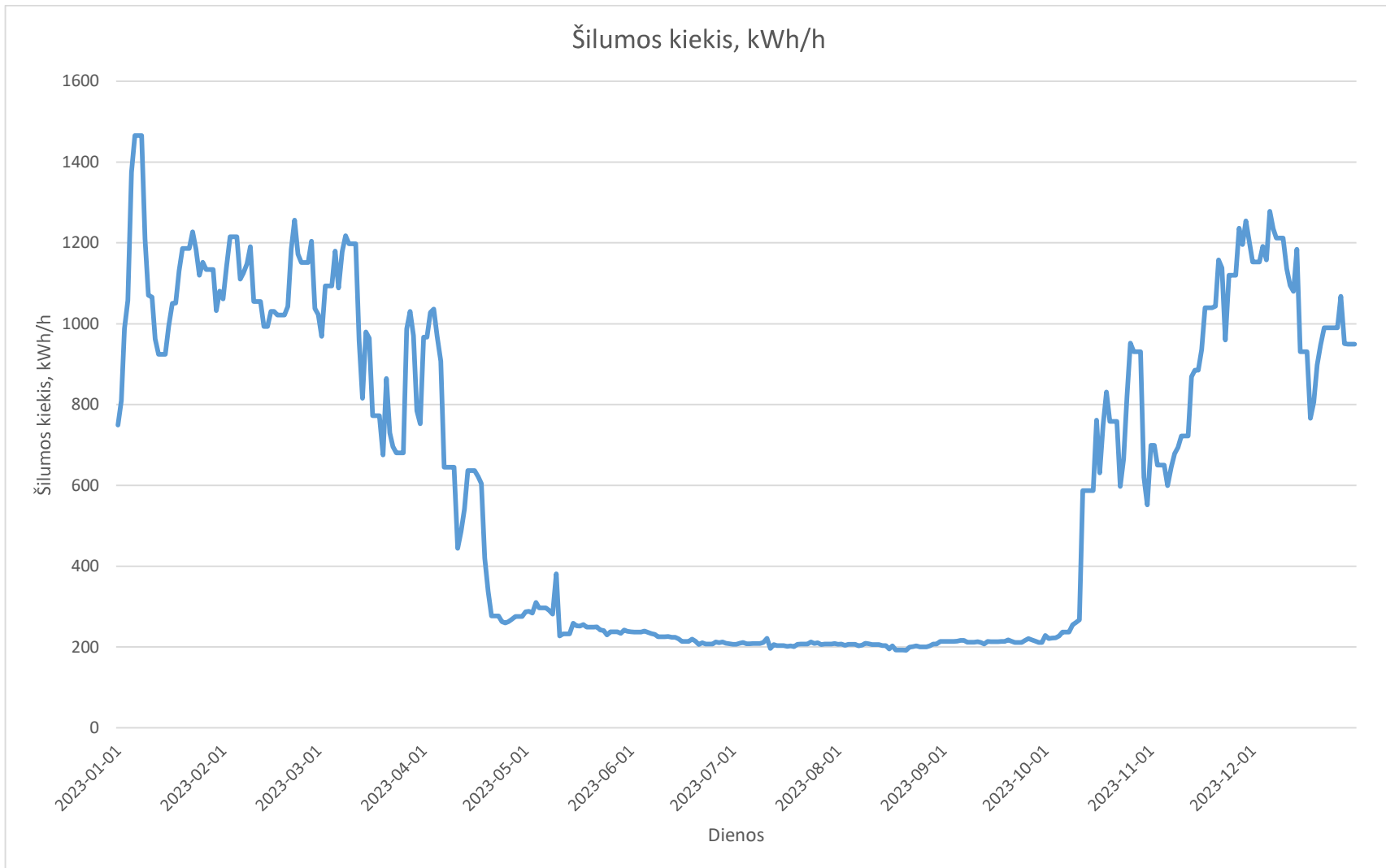
2023m. Ginkūnų katilinės paros vidutinės šilumos gamybos grafikas
