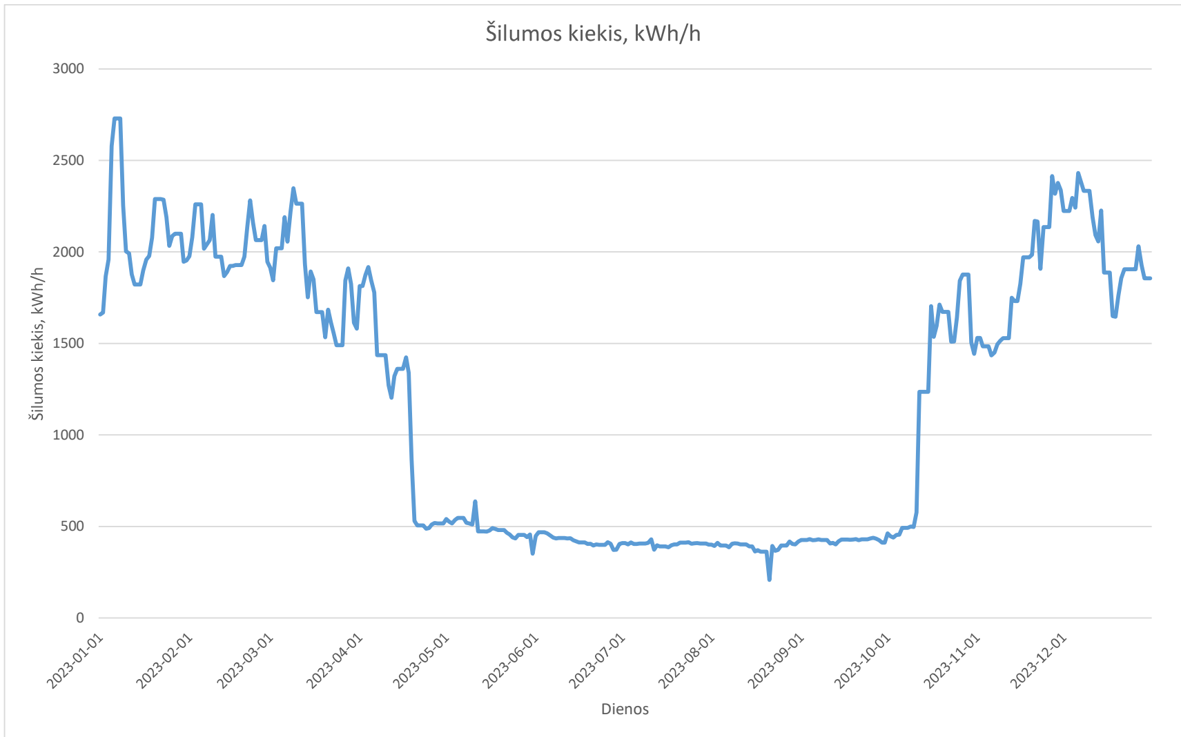
2023m. Daugėlių katilinės paros vidutinės šilumos gamybos grafikas
