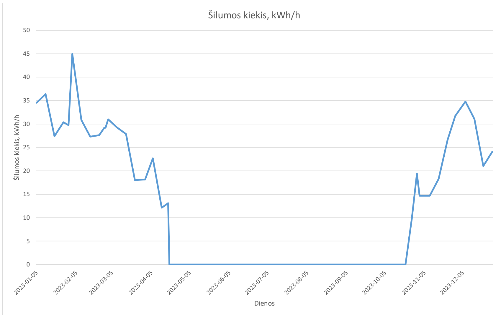
2023m. Basanavičiaus g. katilinės paros vidutinės šilumos gamybos grafikas
