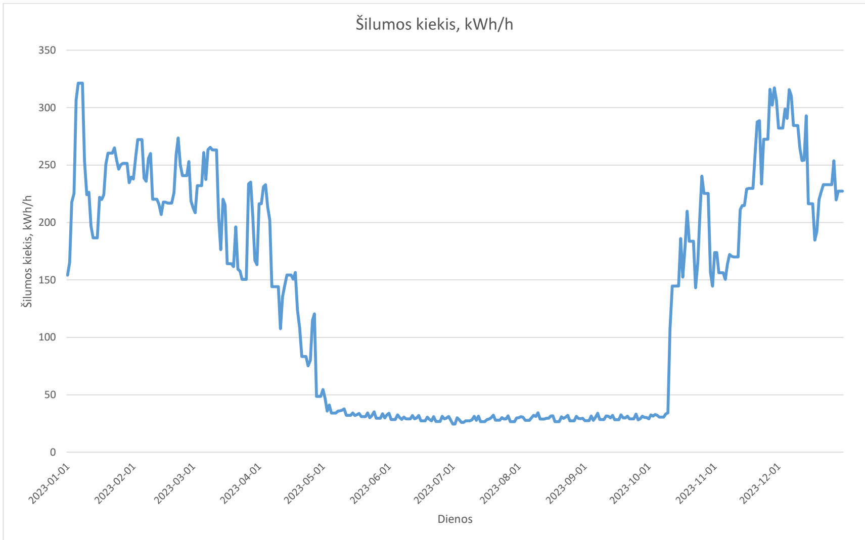
2023m. Aukštelkės katilinės paros vidutinės šilumos gamybos grafikas
